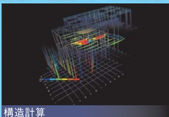
構造計算
